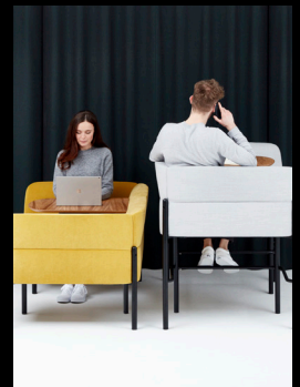
Divide & Conquer
